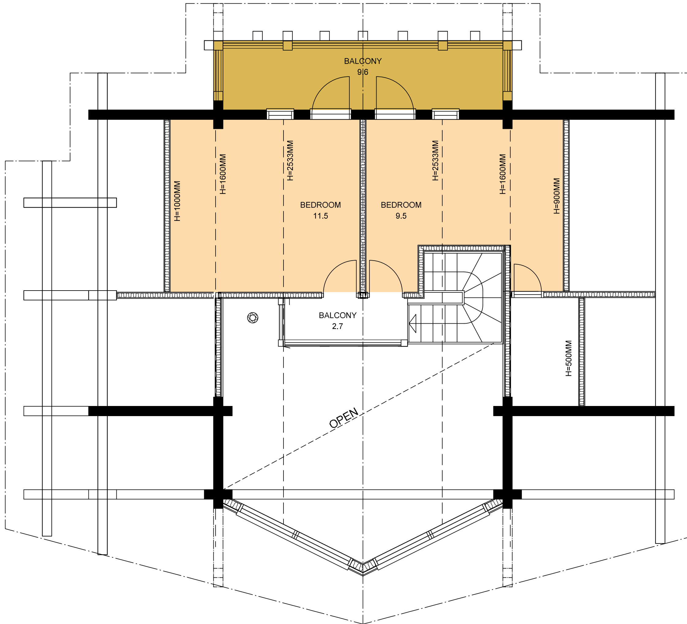
2 FLOOR 1;50 PROJECT H2-107
