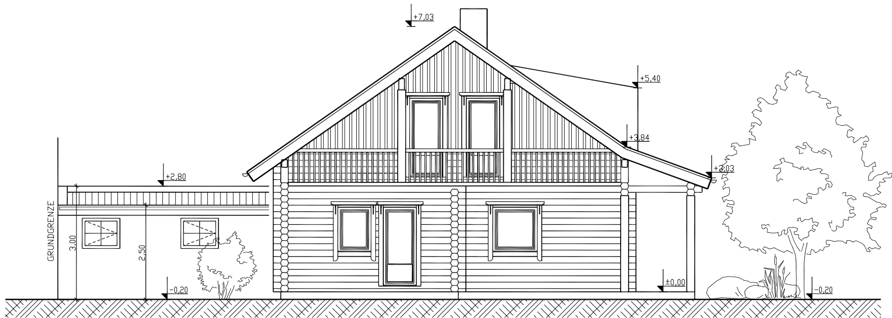
WESTANSICHT
