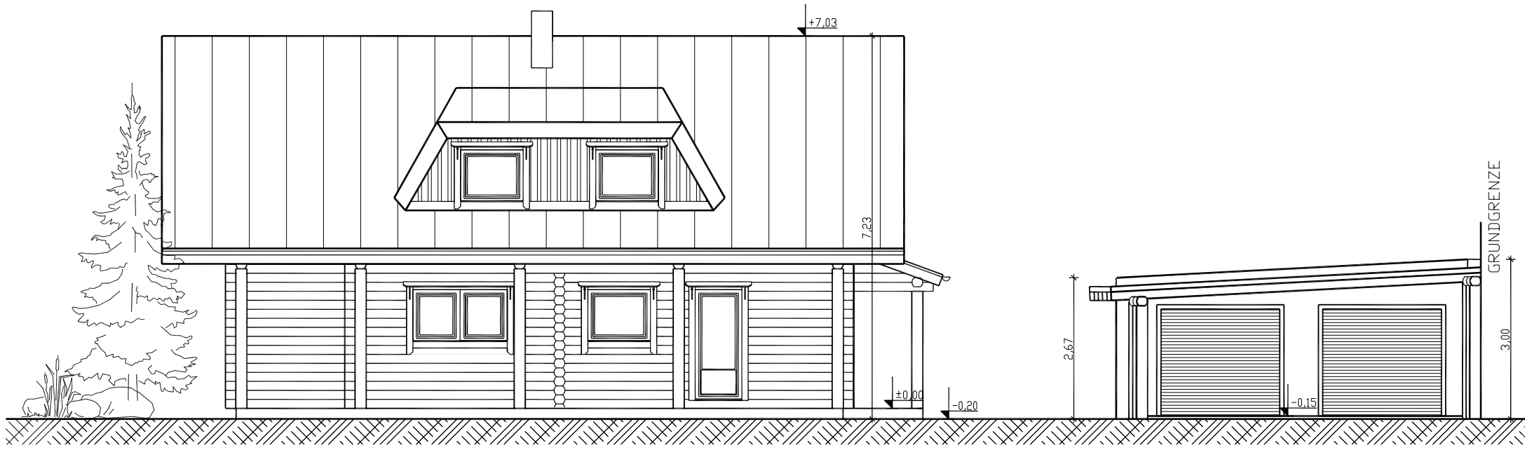
SÜDANSICHT
